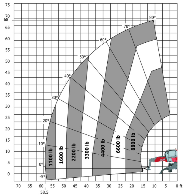
Machine sur stabilisateurs abaissés avec potence 4000 kg (Impérial)
