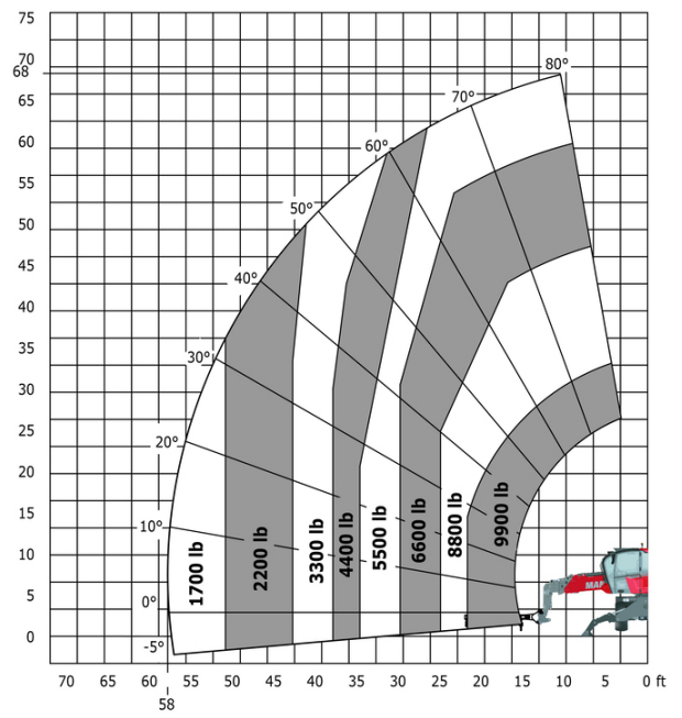
Machine sur stabilisateurs abaissés avec crochet 5000 kg (Impérial)
