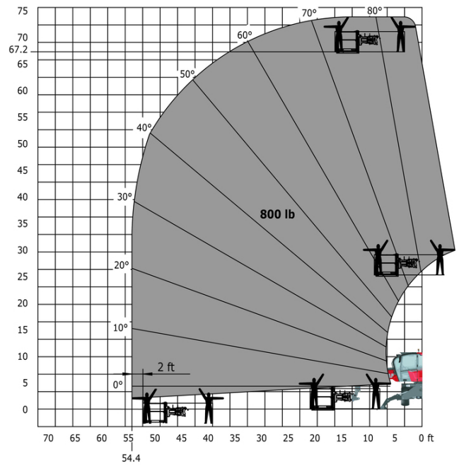
Machine sur stabilisateurs abaissés avec nacelle 365 kg Impérial
