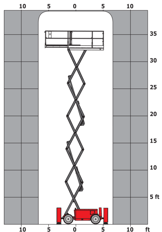
Abaque de charge pour nacelle (impérial)
